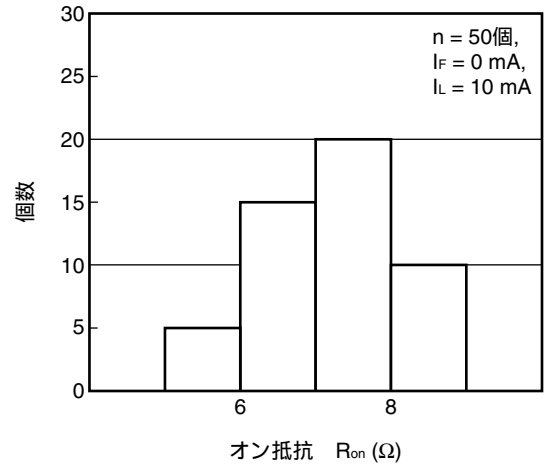
オン抵抗 (N.C.) 分布
