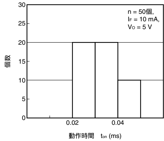
動作時間 (N.C.) 分布
