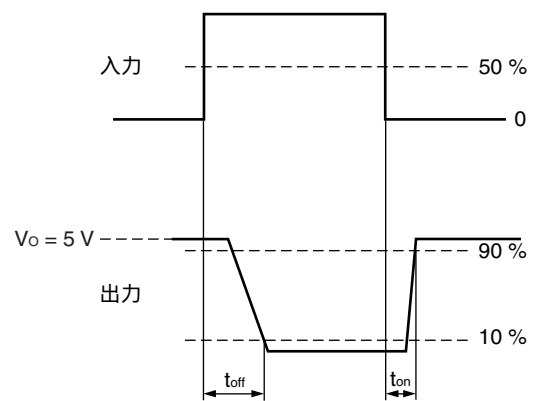
N.C. (7, 8番ピン間)
