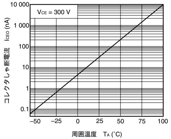
コレクタしや断電流 vs. 周囲温度
