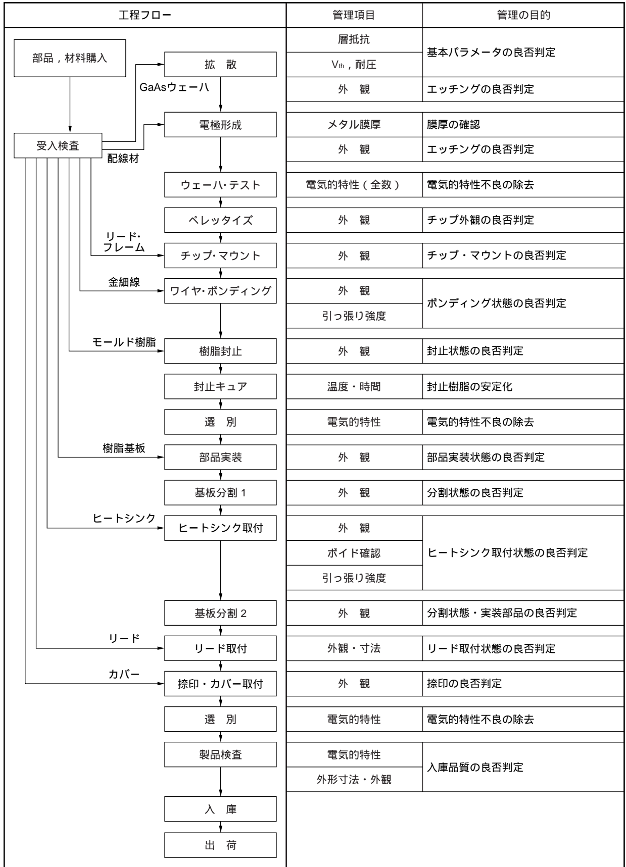
図 2 - 1 CATV 用モジュール製造工程管理フローチャート例
