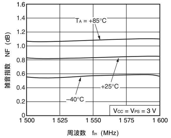
雑音指数 vs. 周波数
