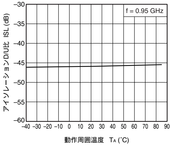
アイソレーションD/U比 vs. 動作周囲温度
