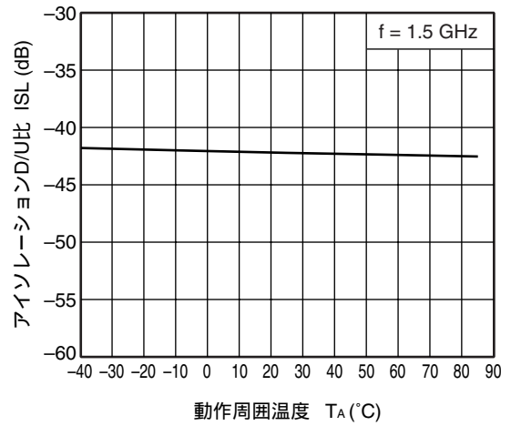
アイソレーションD/U比 vs. 動作周囲温度
