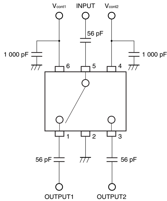
評価回路図 ( V_{cont} = 2.8 V/0 V , DC カット・コンデンサ = 56 pF)
