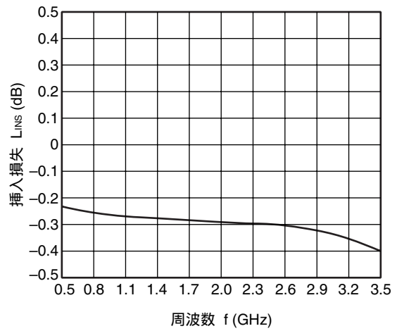
INPUT-OUTPUT2 挿入損失 vs. 周波数
