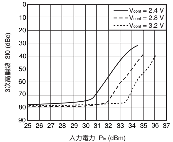
3次高調波 vs. 入力電力の電圧依存性
