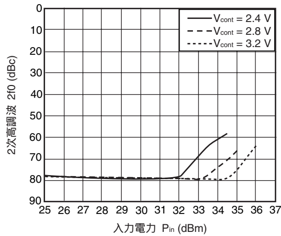
2次高調波 vs. 入力電力の電圧依存性
