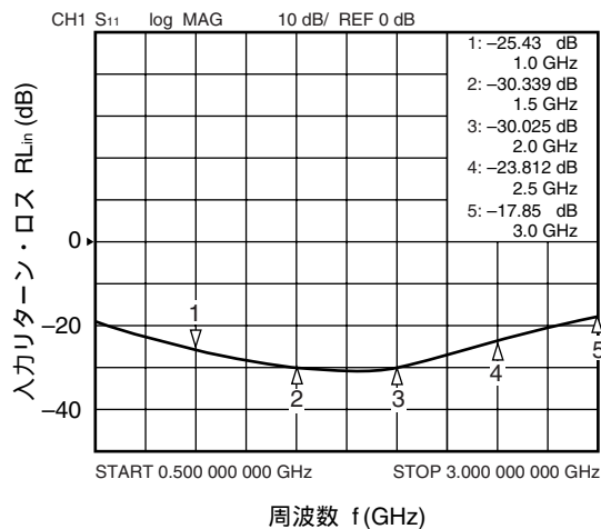
入力リターン・ロス vs. 周波数
