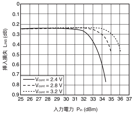
挿入損失 vs. 入力電力の電圧依存性
