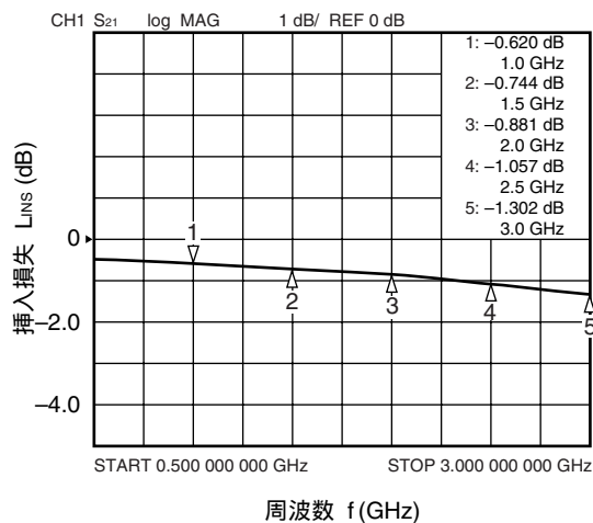
挿入損失 vs. 周波数
