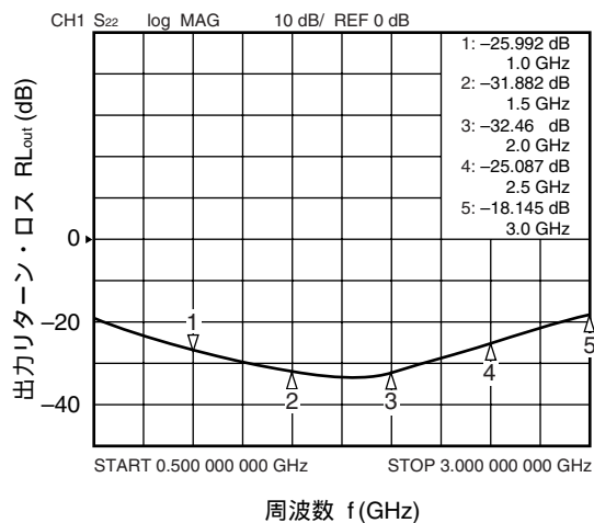
出力リターン・ロス vs. 周波数
